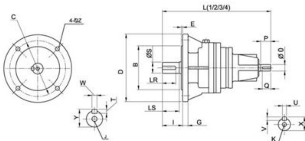
尺寸規格表 DIM.TABLE (mm)
