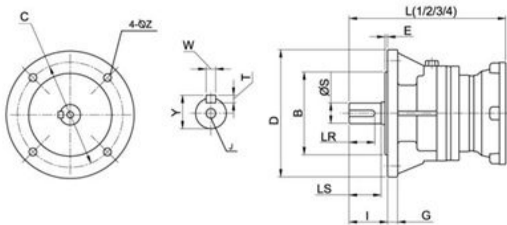
尺寸規格表 DIM.TABLE (mm)
