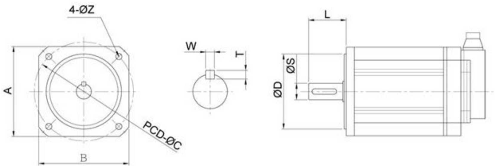
伺服馬達尺寸表 Servo Motor Dimension
